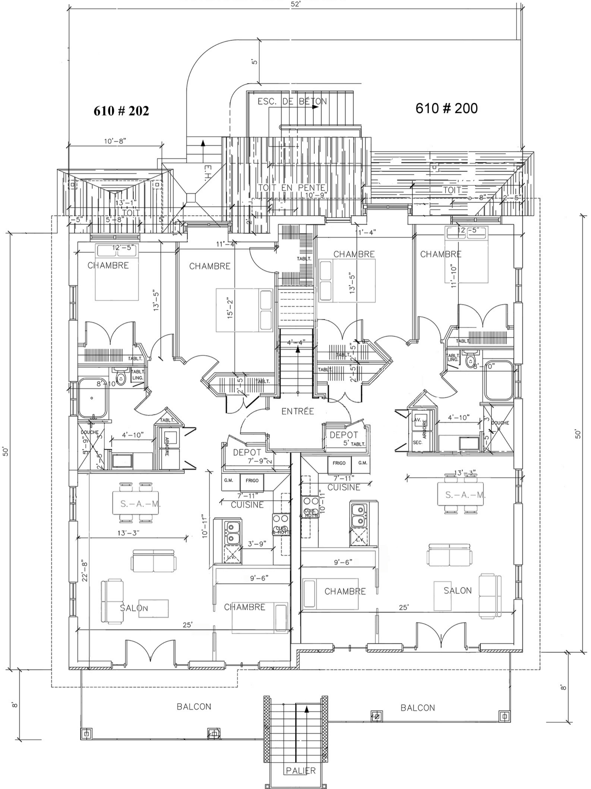
PLAN NIVEAU ÉTAGE-2
